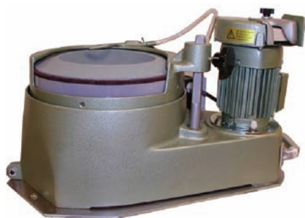
TMP Slipemaskin G 91 (stor) Med liggende sten, filtskive og lukket vannkjøling. Spenning: 230/400V - 3 fas, 50Hz Vekt: 37kg
